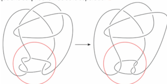
El nudo de Conway (derecha) y el nudo de Kinoshita-Terasaka (izquierda) son mutantes, es decir, uno puede obtenerse a partir del otro girando el círculo rojo.
