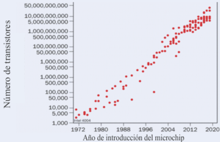
Gráfica descriptiva de la Ley de Moore. (Adaptada de wikipedia.org/wiki/Transistor_count). Original de Hannah Ritchie and Max Roser).
