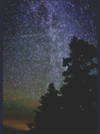
Estrella fugaz y trazos de estrellas en una noche sin Luna.
