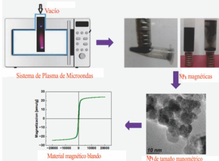
Figura 1. Material magnético fabricado por la técnica de plasma de microondas.
