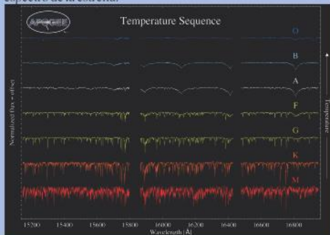
Espectros APOGEE (flujo por unidad de longitud), ordenados en base a su temperatura, siendo la estrella de tipo espectral O la más caliente. Créditos: Steven Majewski y la colaboración SDSS.
